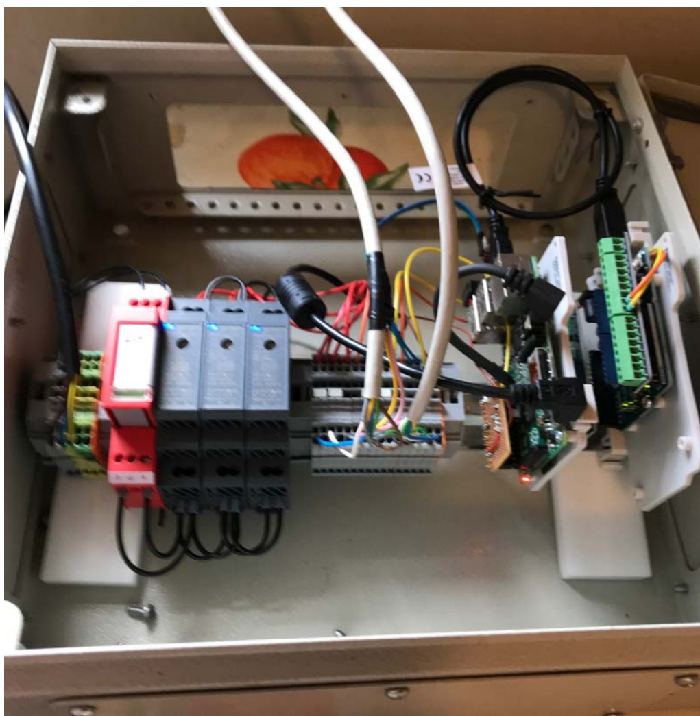
Elektronik Wetterstation.JPG
